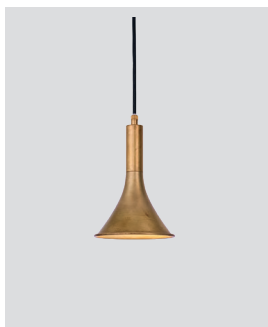
MEGAFON STRAIGHT D. 140 mm H. 195 mm Max 10 W G9 3460-6 Raw brass
